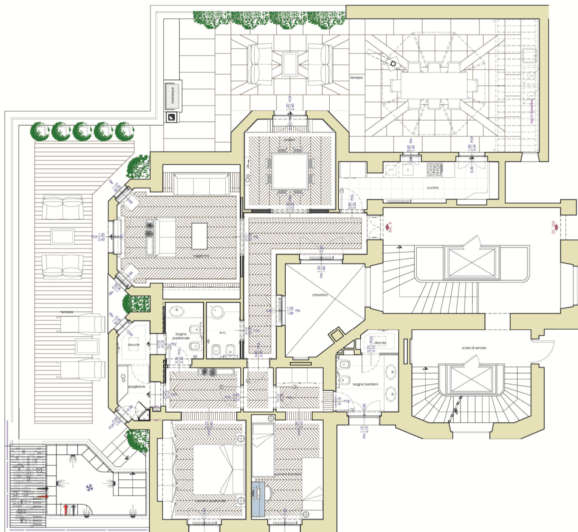
Planimetria attico
